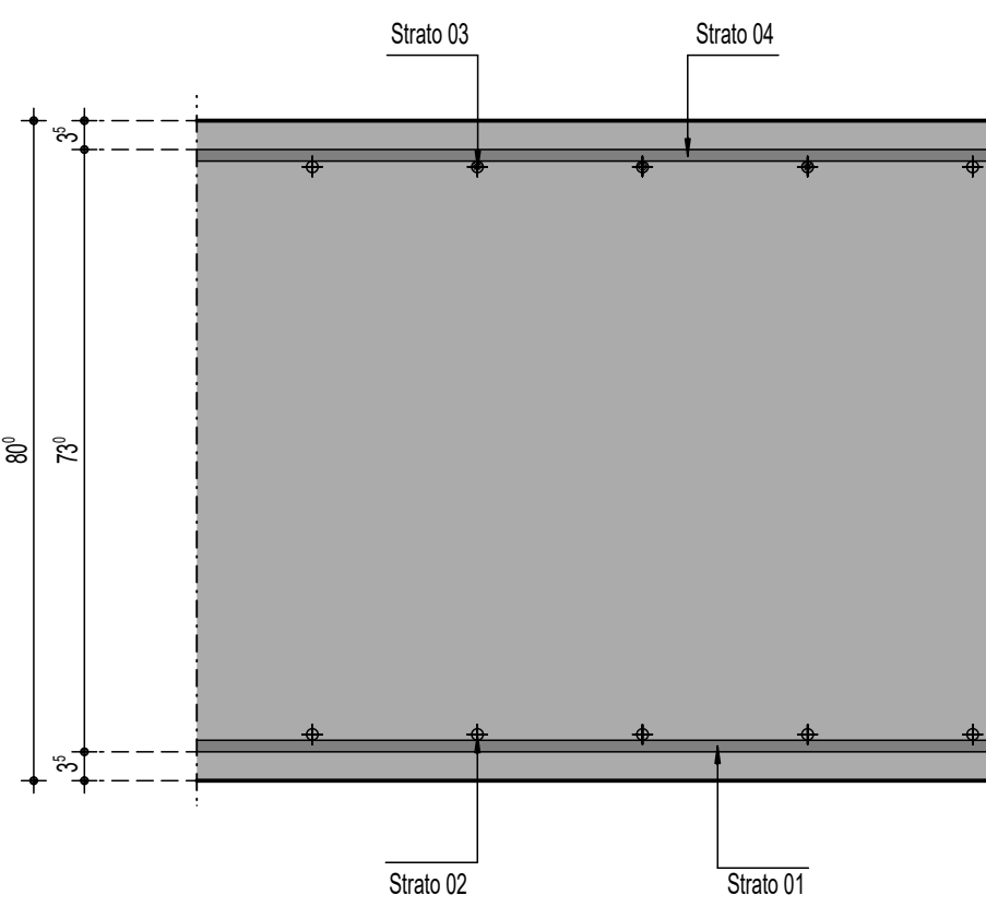
dettaglio STRATI di posa delle ARMATURE - PLATEA STAZIONE PL01
