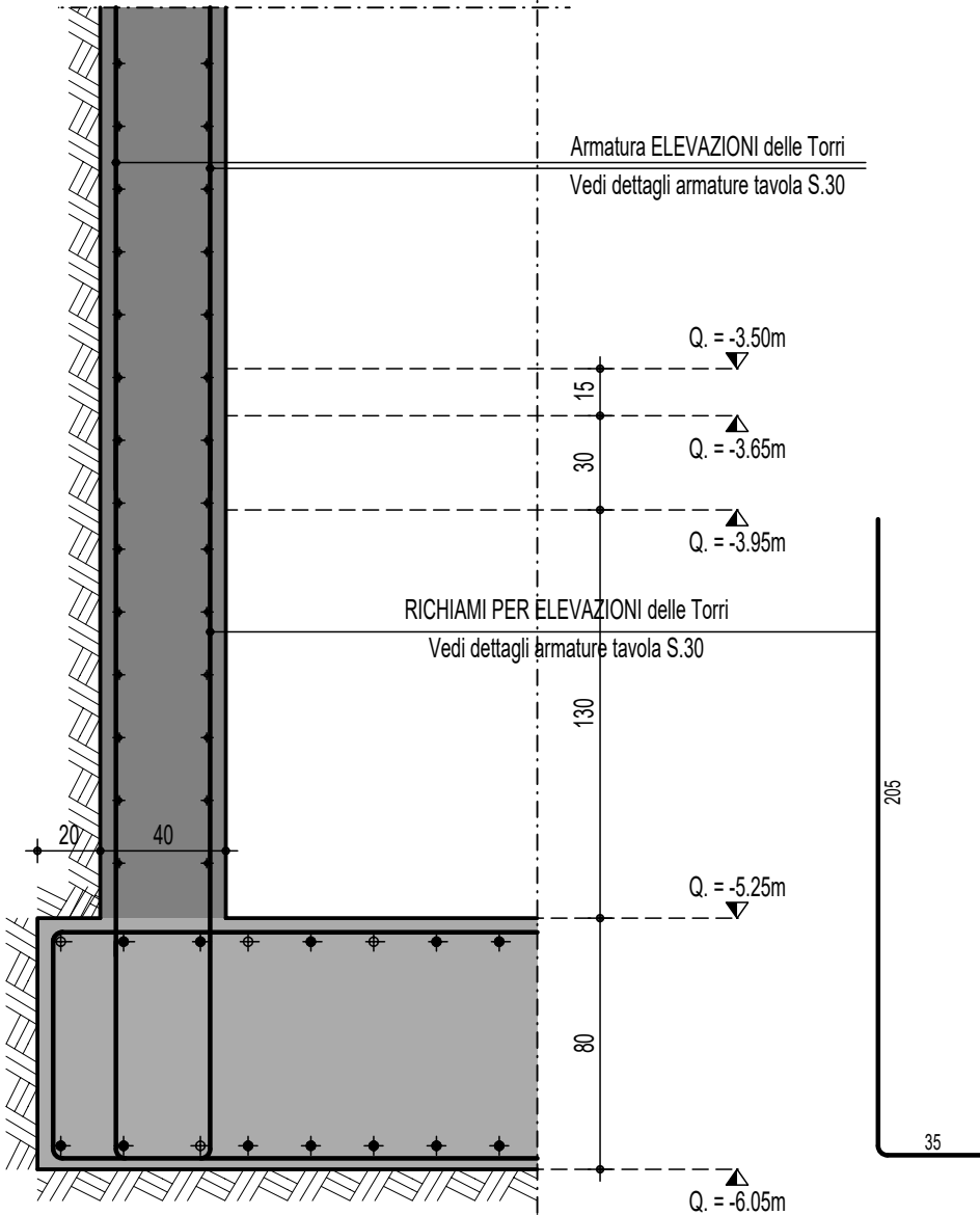
dettaglio TIPO E - ELEVAZIONI TORRI SU PLATEA DI FONDAZIONE E SOLETTA A2 - - scala 1 : 25 -
