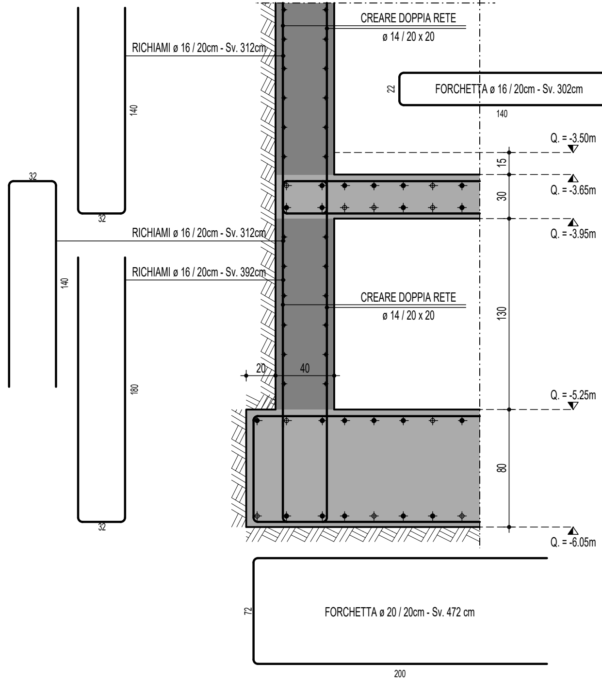
dettaglio TIPO C - NERVATURE DI RINFORZO PLATEA DI FONDAZIONE - - scala 1 : 25 -
