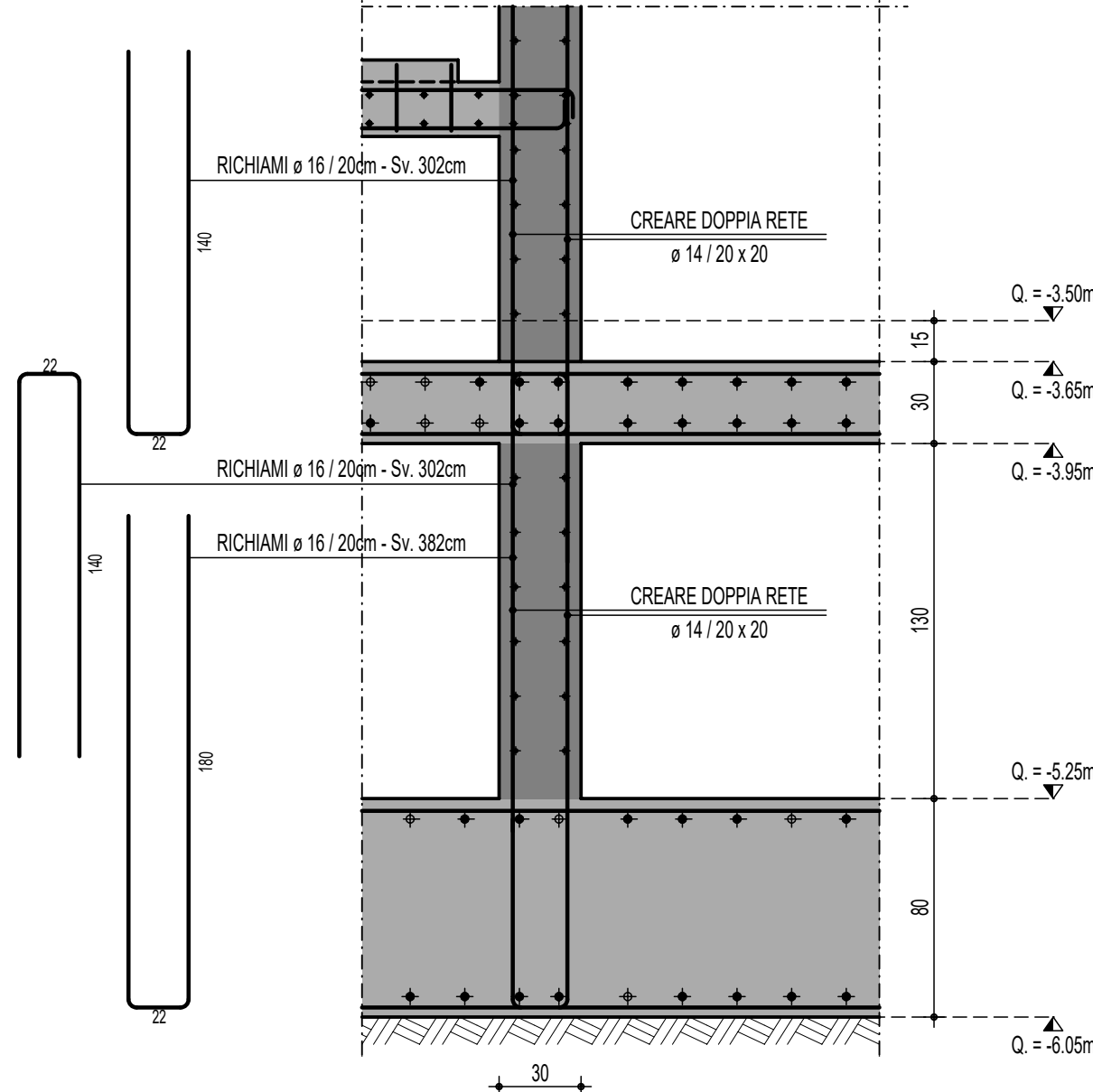
dettaglio STRATI di posa delle ARMATURE - PLATEA STAZIONE PL01
