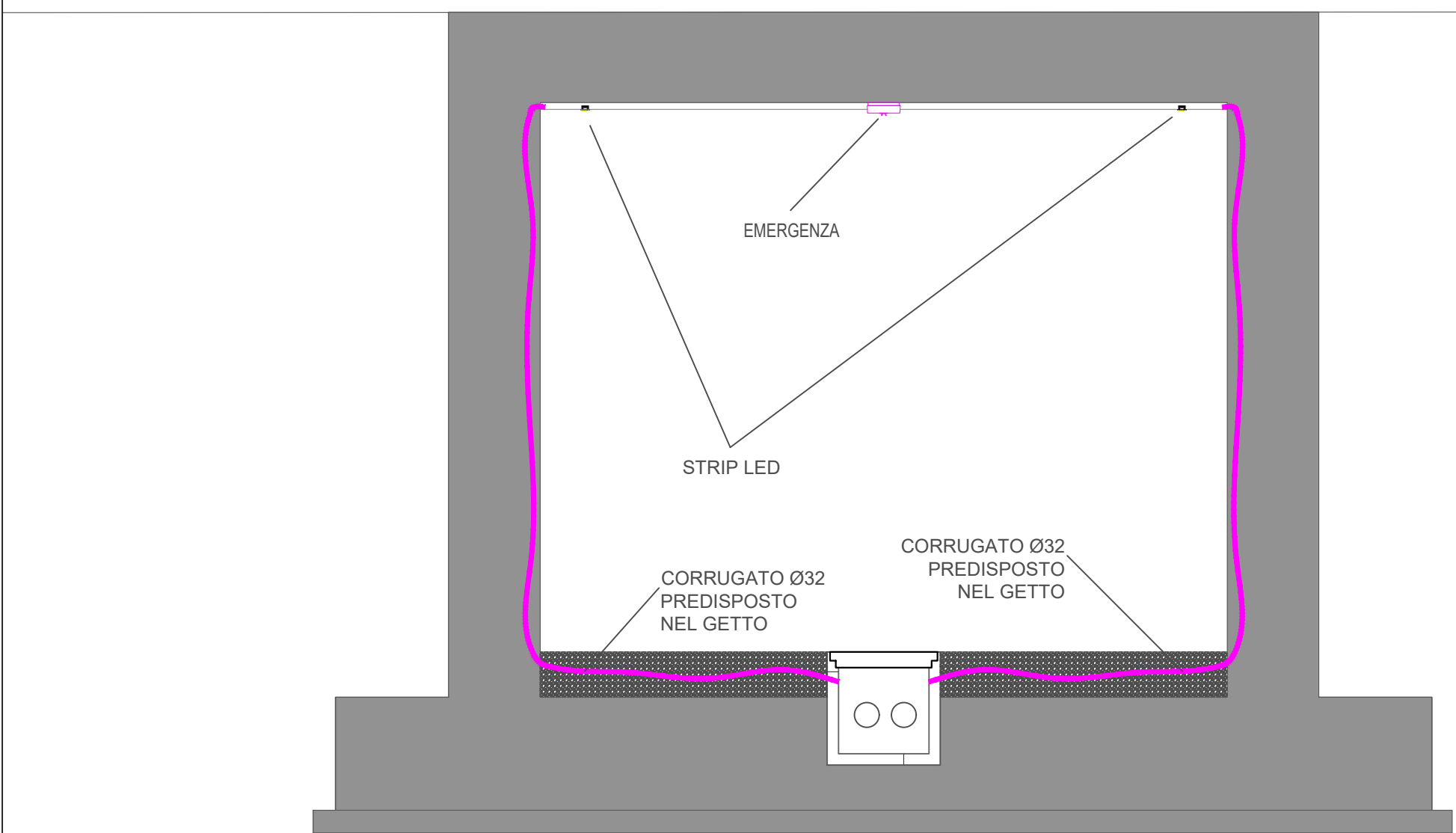
PARTICOLARE DISTRIBUZIONE SOTTOPASSO
