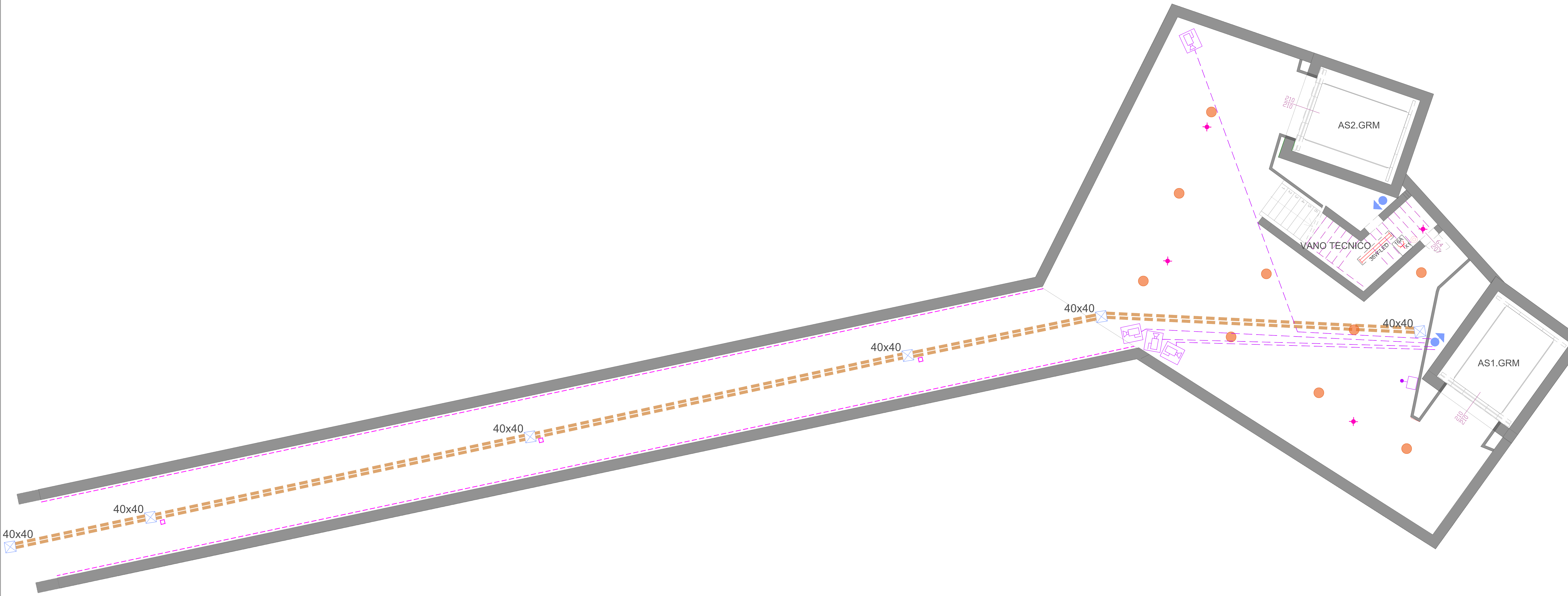
PLANIMETRIA DISTRIBUZIONE ED APPARECCHIATURE QUOTA -3.50m
