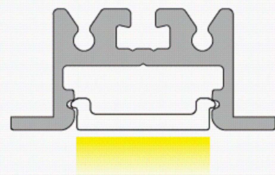
PARTICOLARE LAMPADA EMERGENZA SOTTOPASSO
