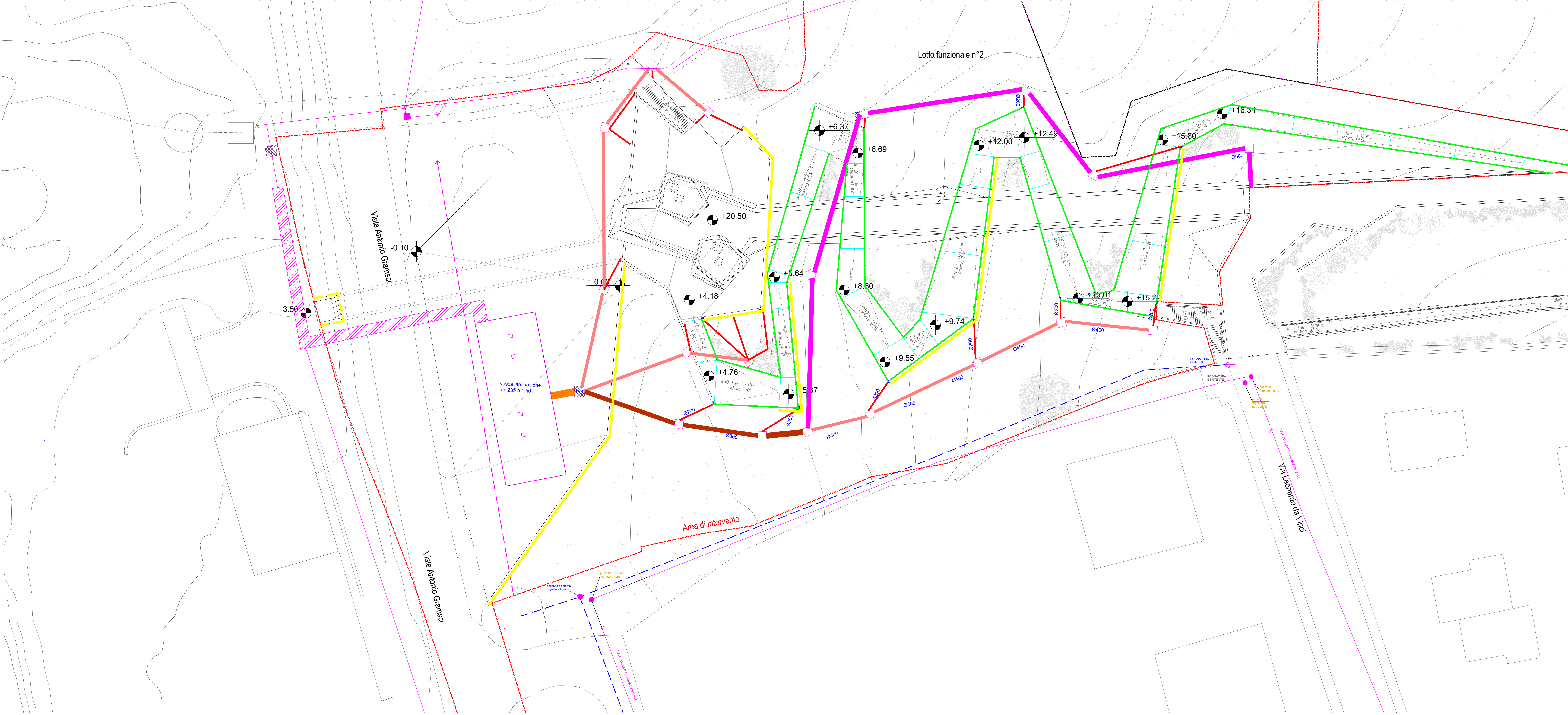
PLANIMETRIA Scala 1:200
