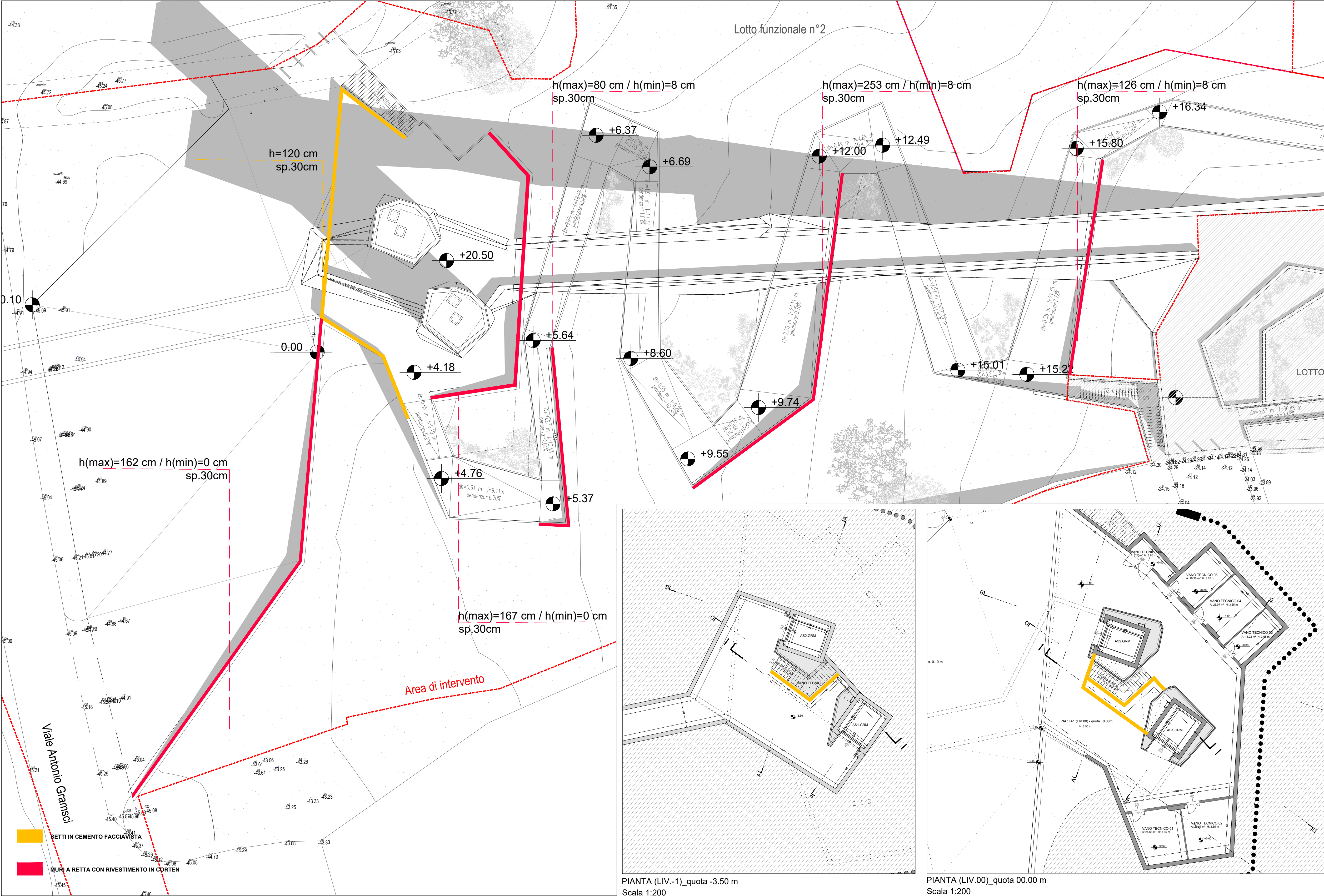
PLANIMETRIA GENERALE Scala 1:200
