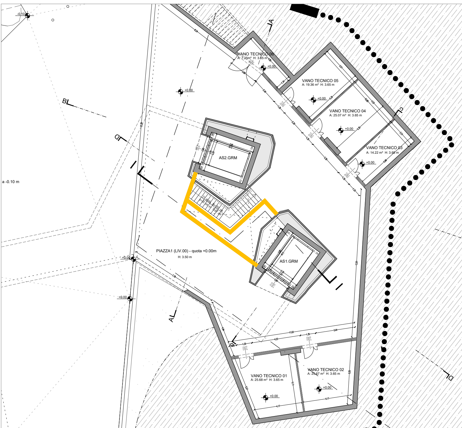
PIANTA (LIV.00)_quota 00.00 m Scala 1:200
