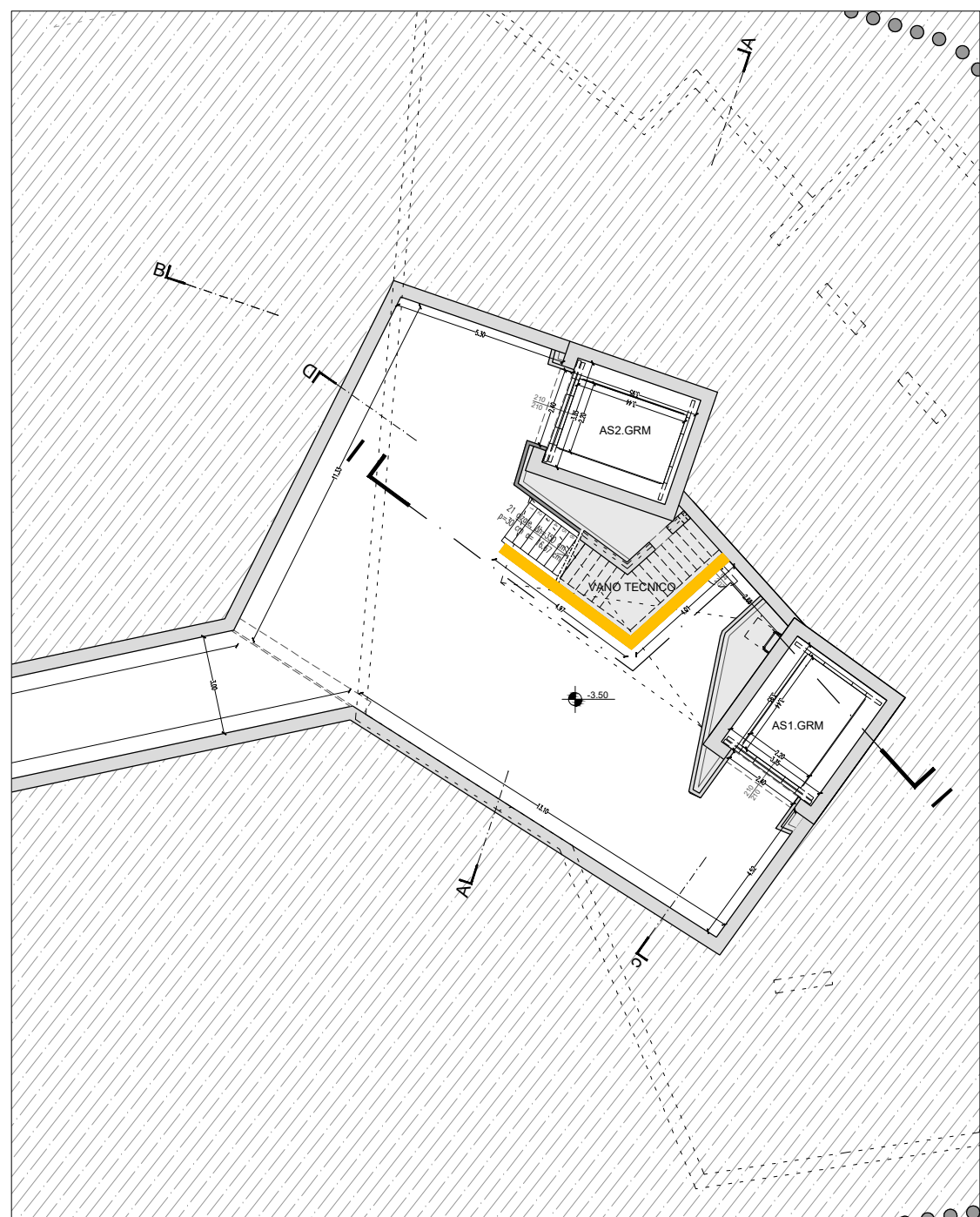
PIANTA (LIV.-1)_quota -3.50 m Scala 1:200
