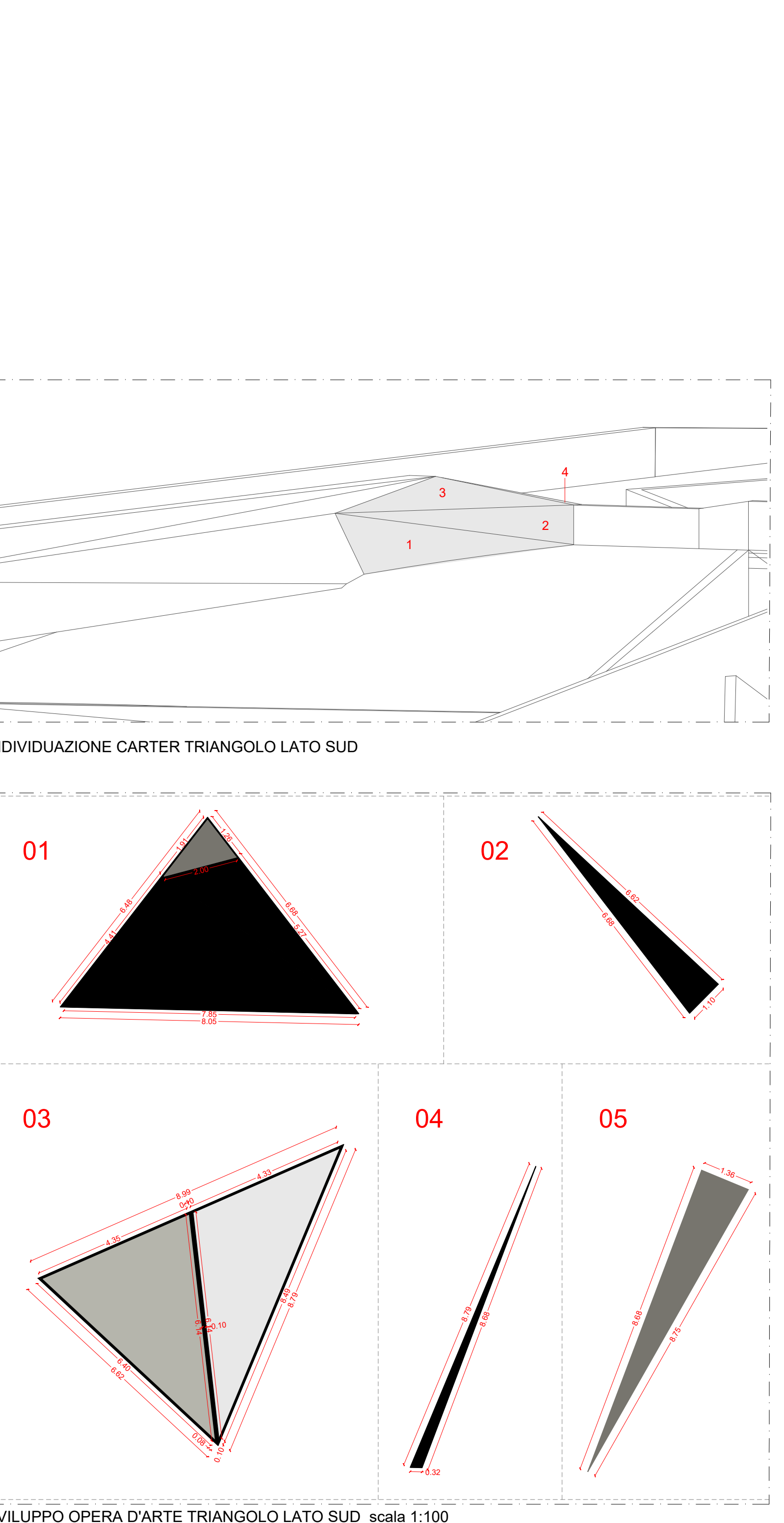
SVILUPPO OPERA D'ARTE TRIANGOLO LATO SUD scala 1:100
