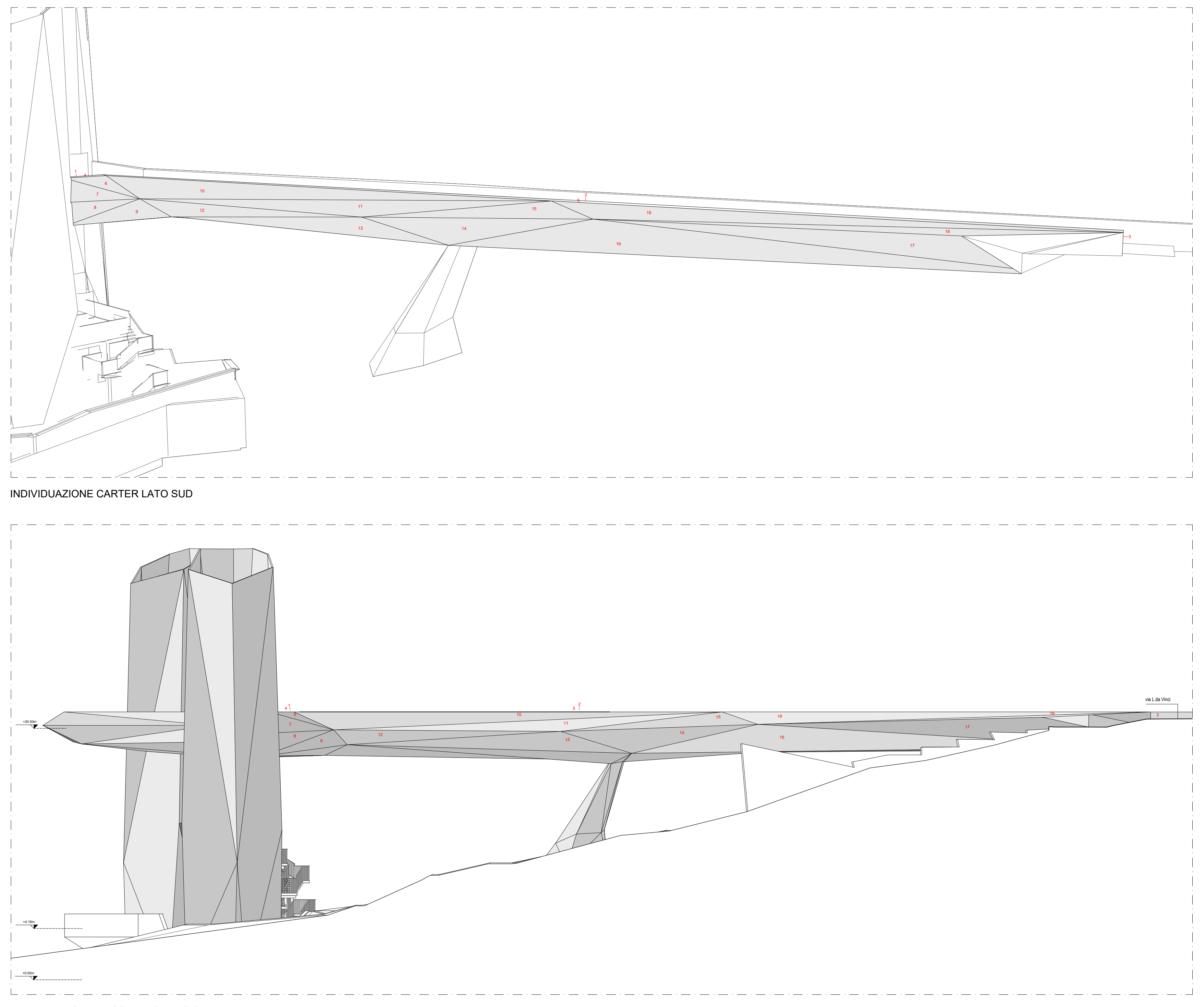
INDIVIDUAZIONE PROSPETTO LATO SUD scala 1:100
