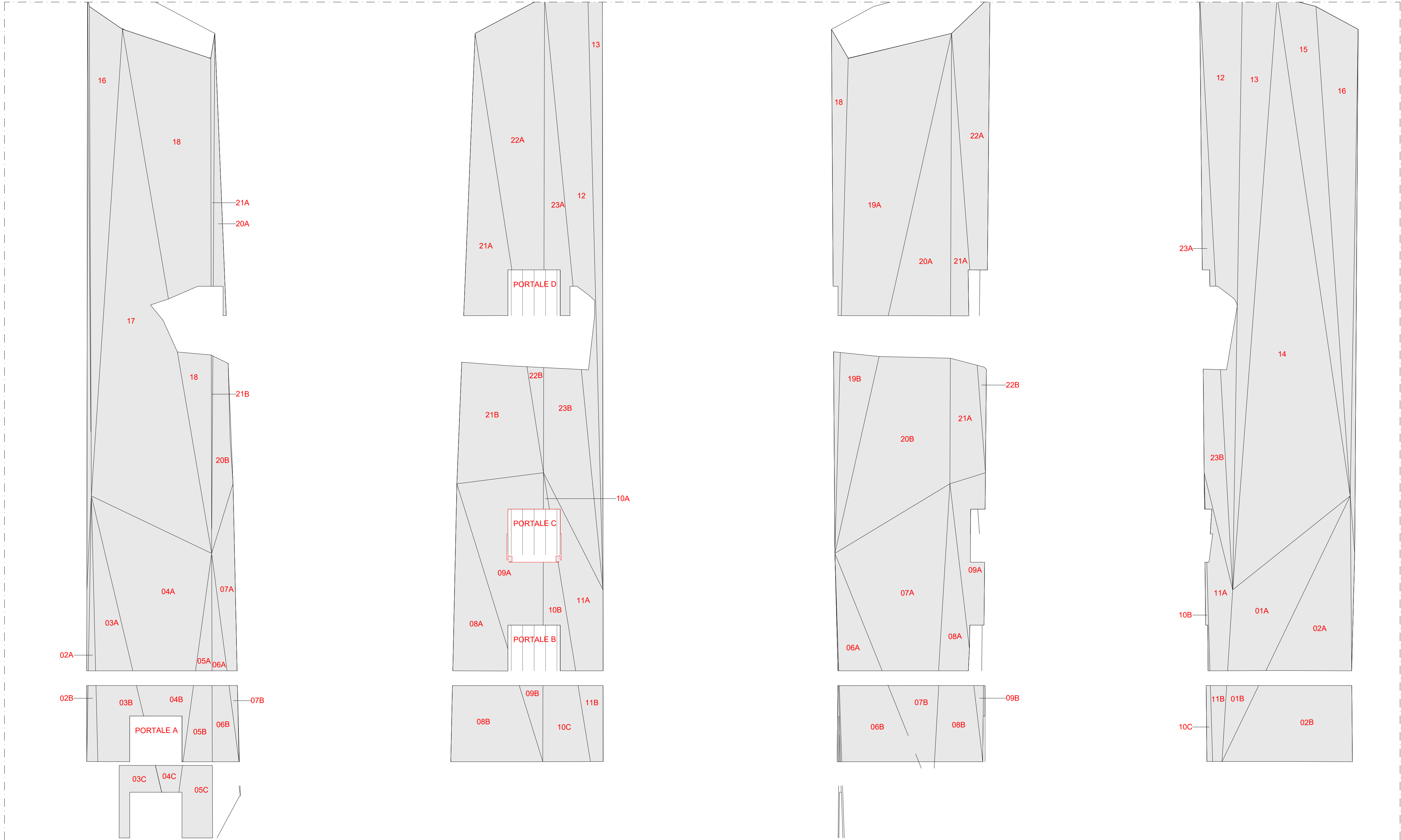
PROSPETTO NORD - OVEST_TORRE A VALLE GRAMSCI 2 Scala 1:100
