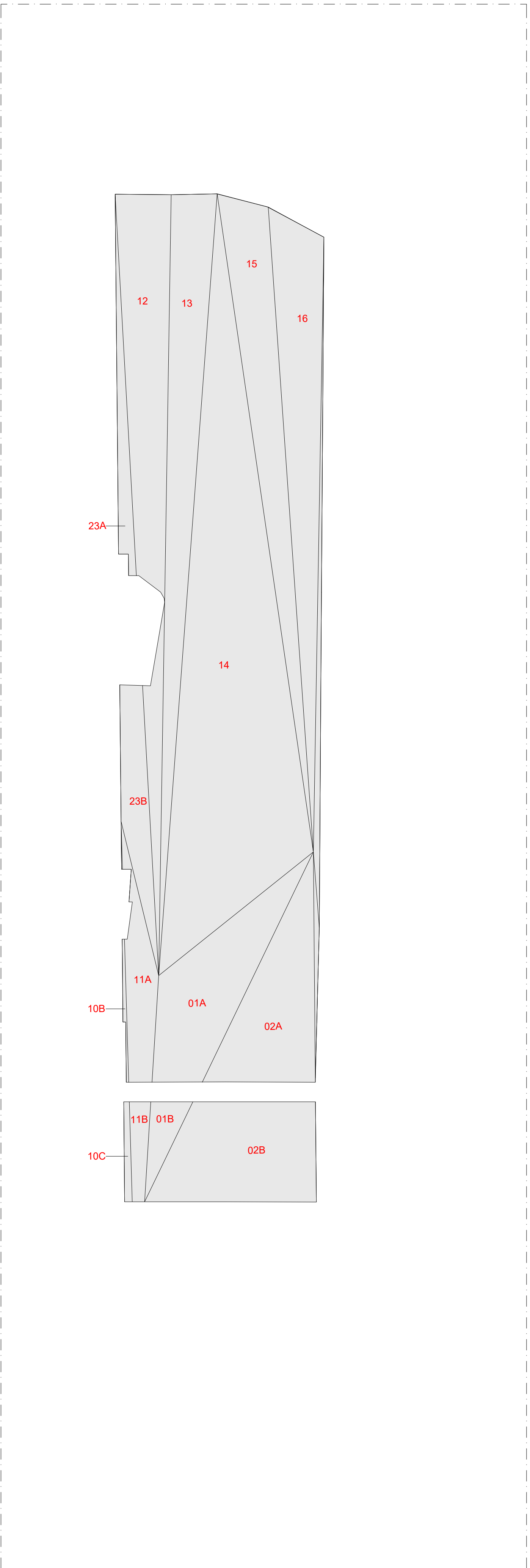
PROSPETTO NORD - EST_TORRE A VALLE GRAMSCI 2 Scala 1:100
