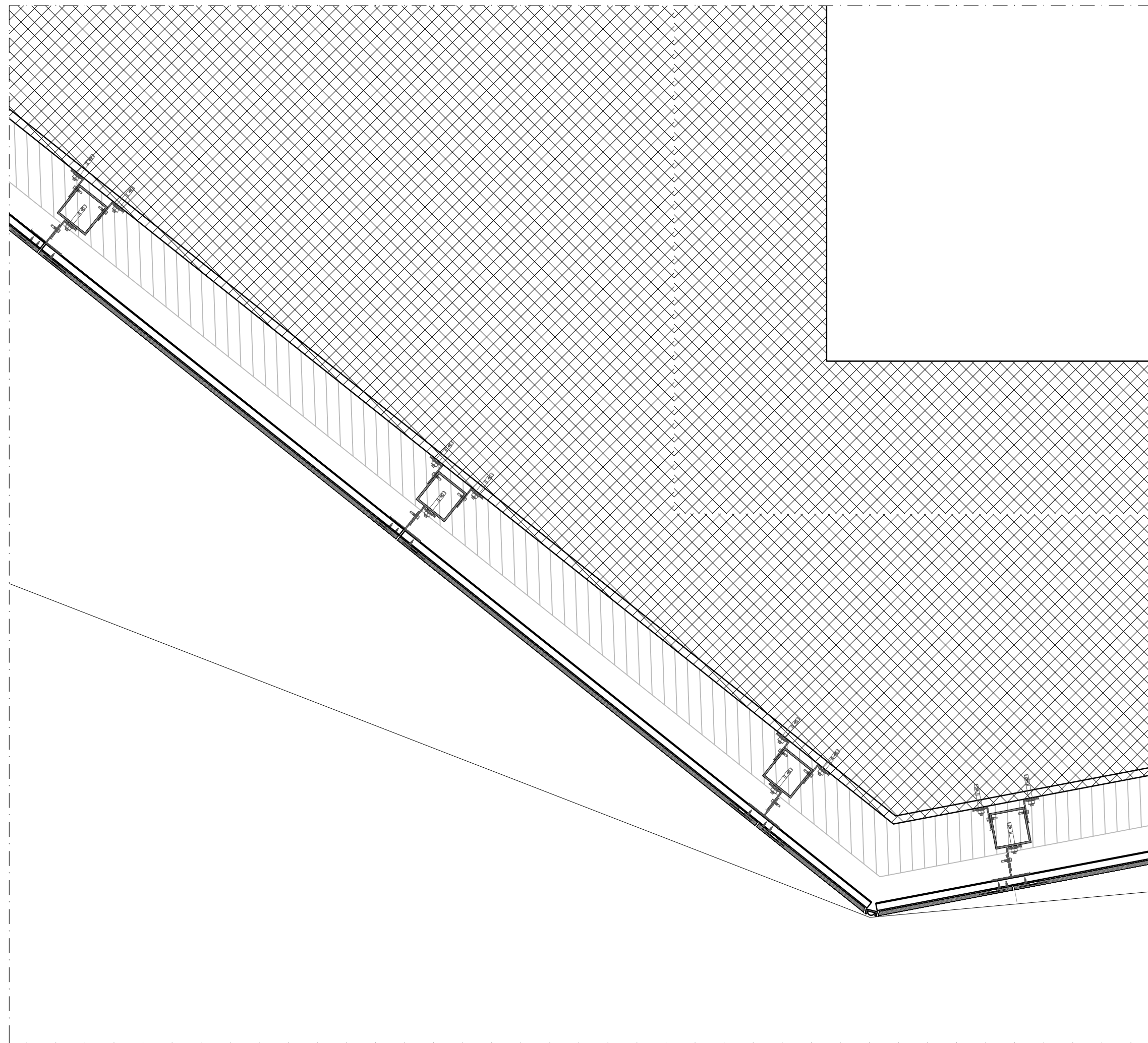
DETTAGLIO COSTRUTTIVO 3 - Pianta Scala 1:10
