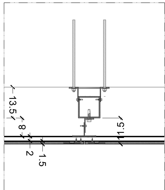
DETTAGLIO COSTRUTTIVO - Pianta Scala 1:10
