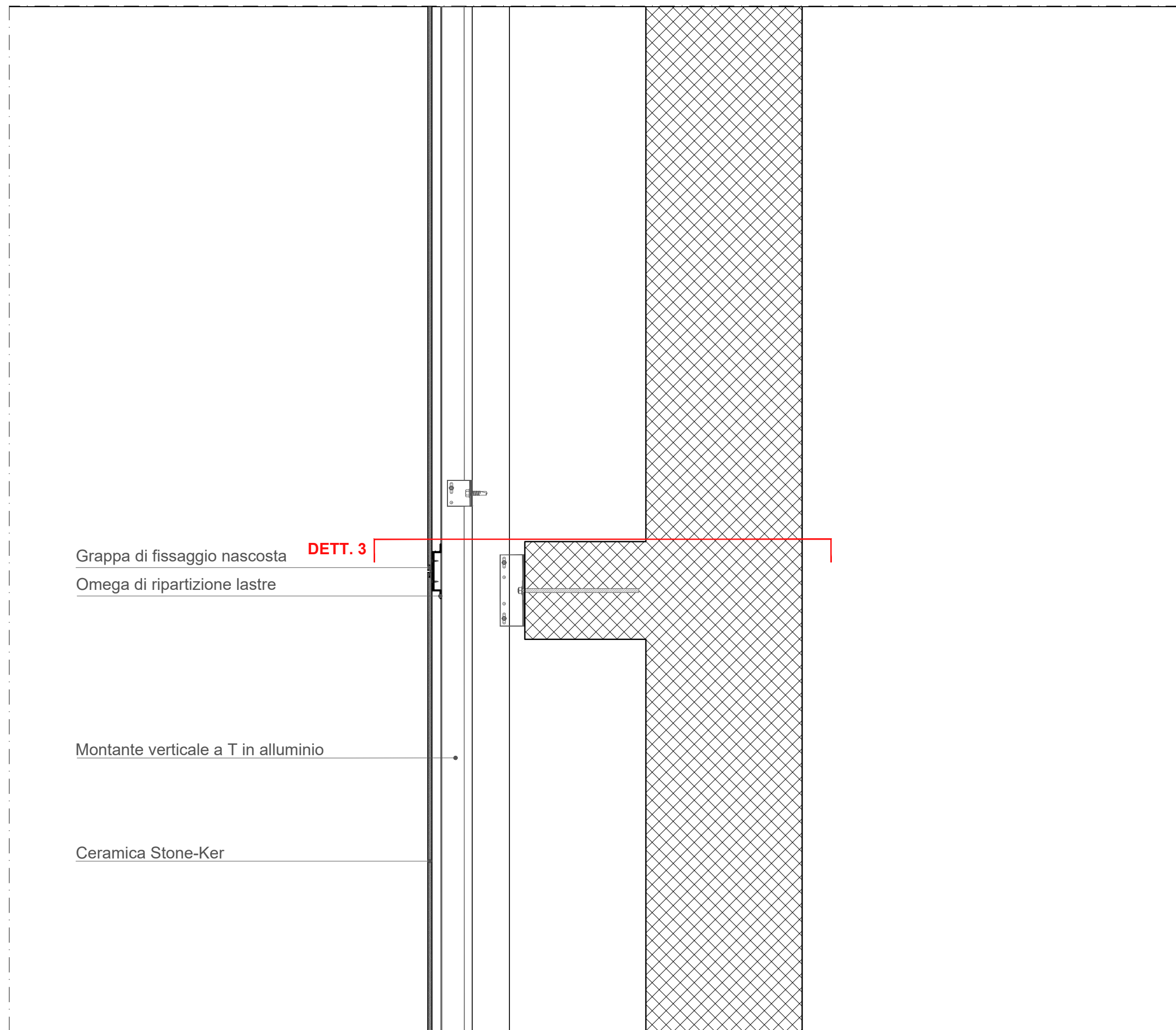
DETTAGLIO COSTRUTTIVO 1 - Sezione Scala 1:10
