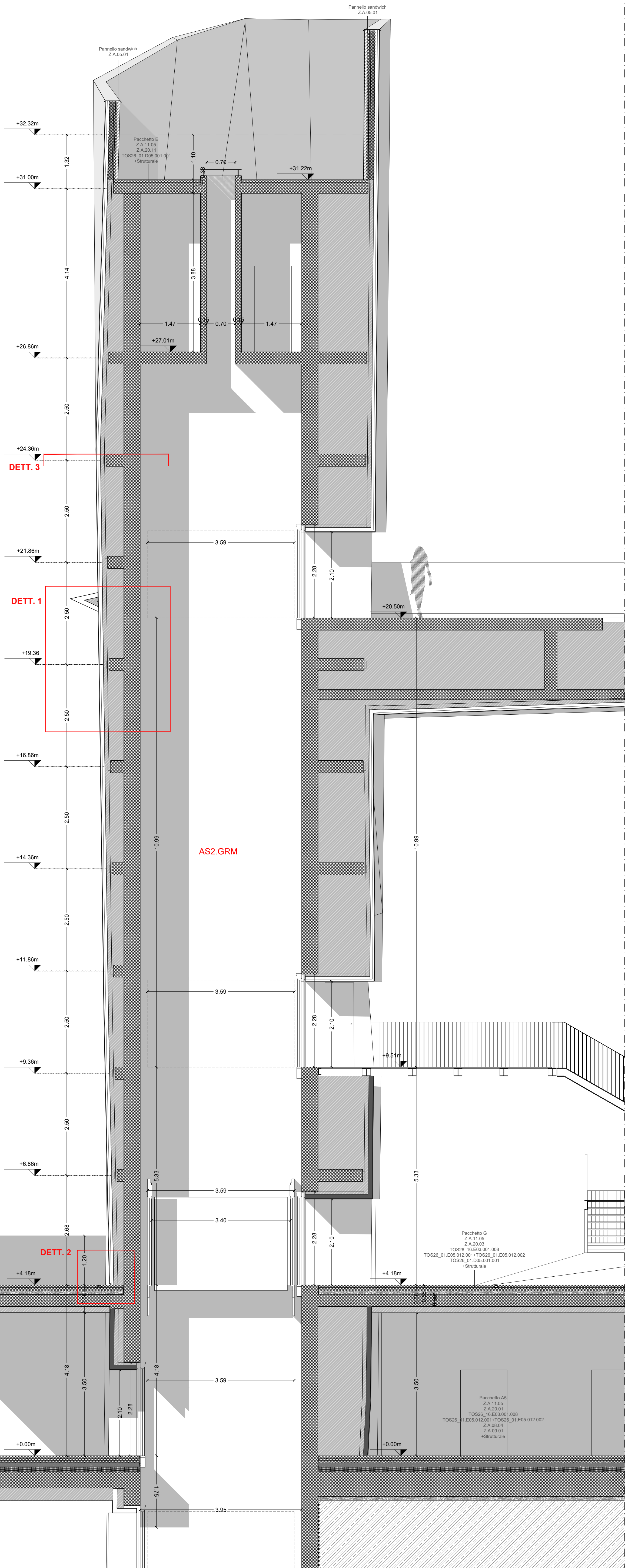
DETTAGLIO COSTRUTTIVO 1 - Sezione Scala 1:10
