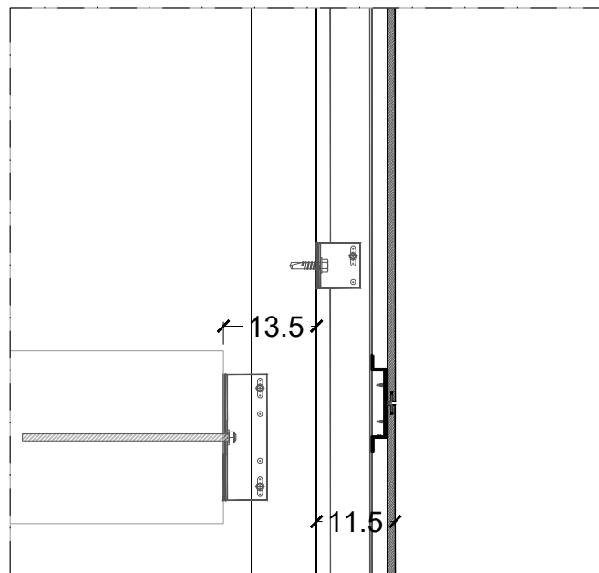
DETTAGLIO COSTRUTTIVO - Sezione Scala 1:10
