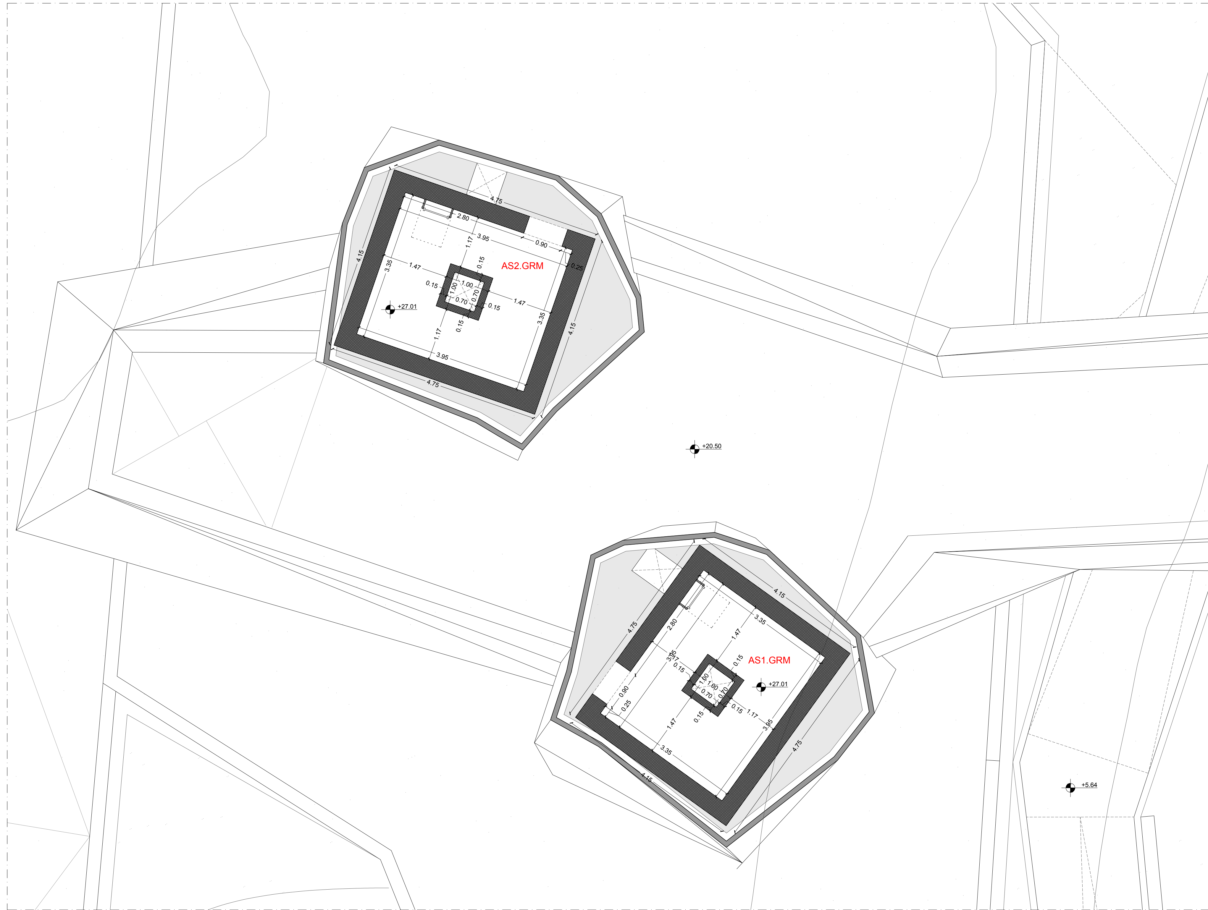
PIANTA (LIV.04)_quota 27.01 m Scala 1:100
