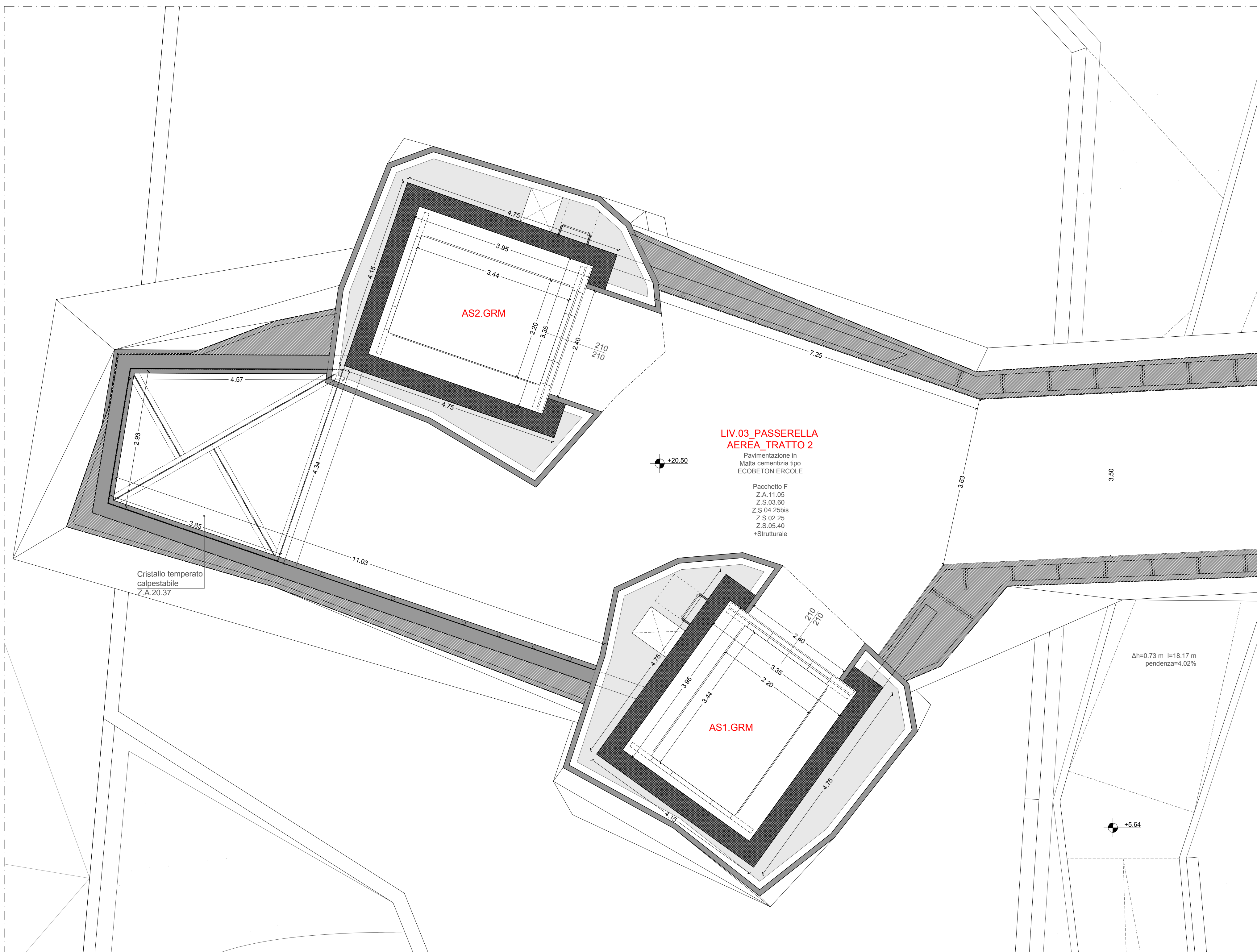
PIANTA (LIV.03)_quota 20.50 m Scala 1:100
