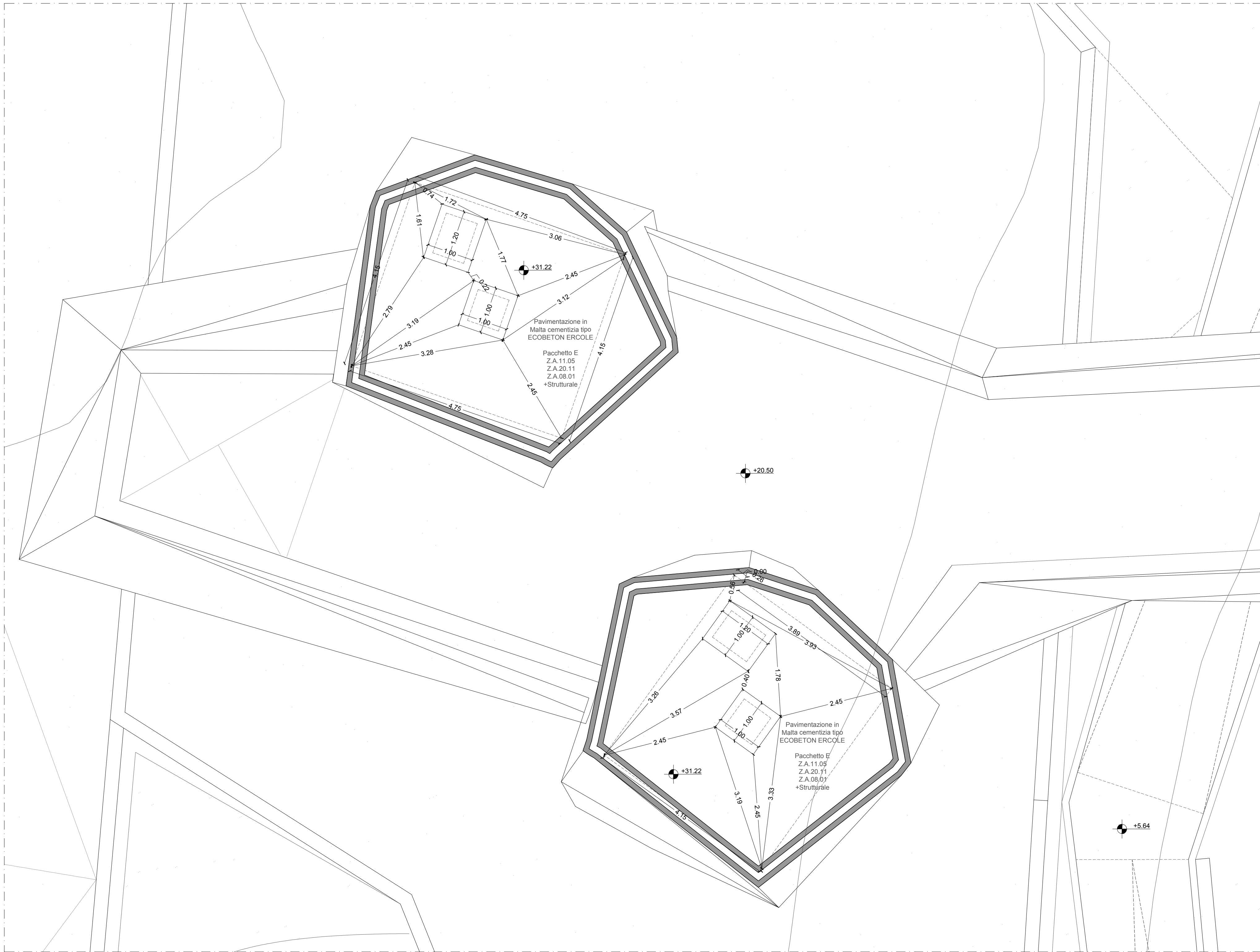
PIANTA (LIV.05)_quota 31.22 m Scala 1:100
