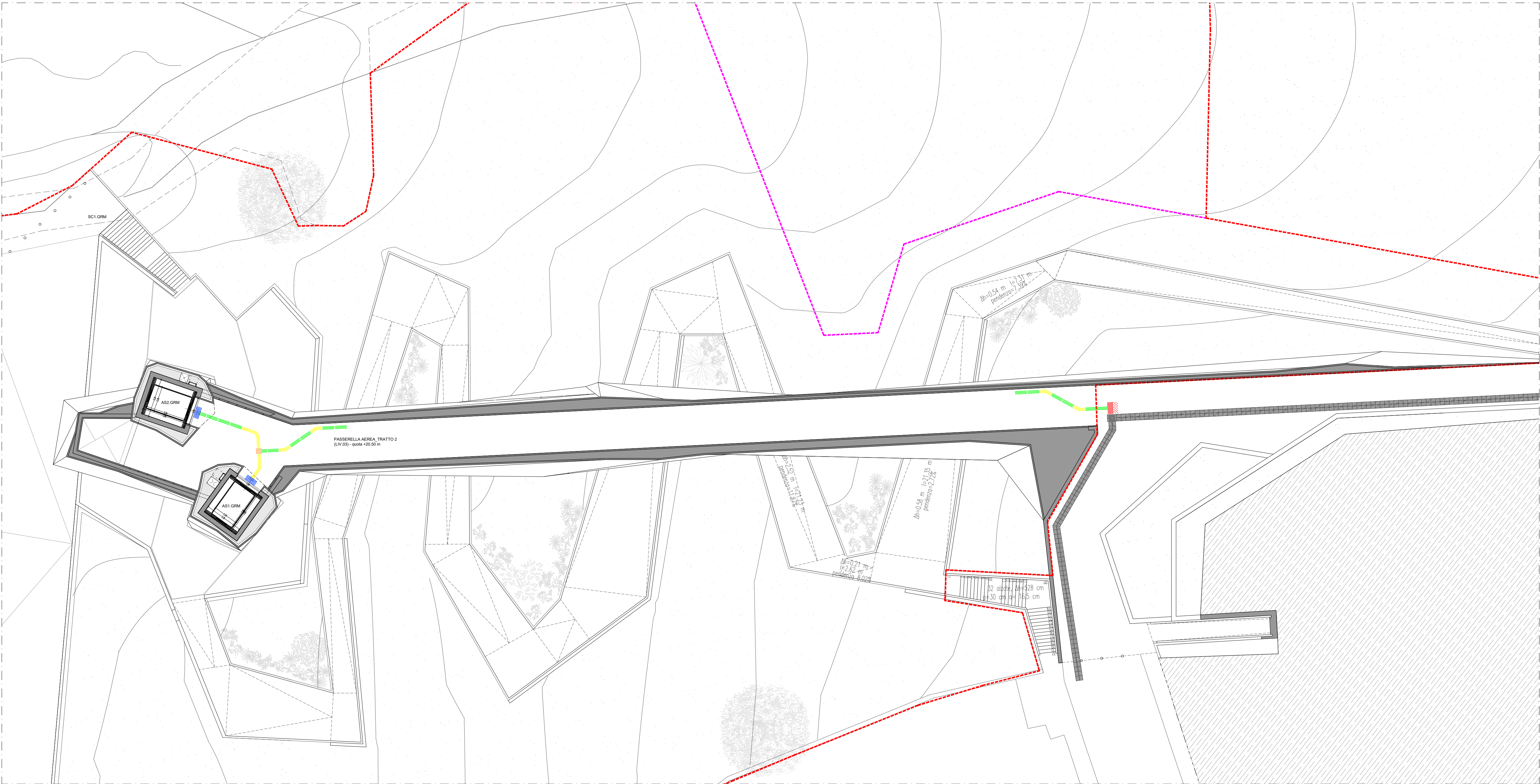
PIANTA (LIV.03)_quota 20.50 m Scala 1:200
