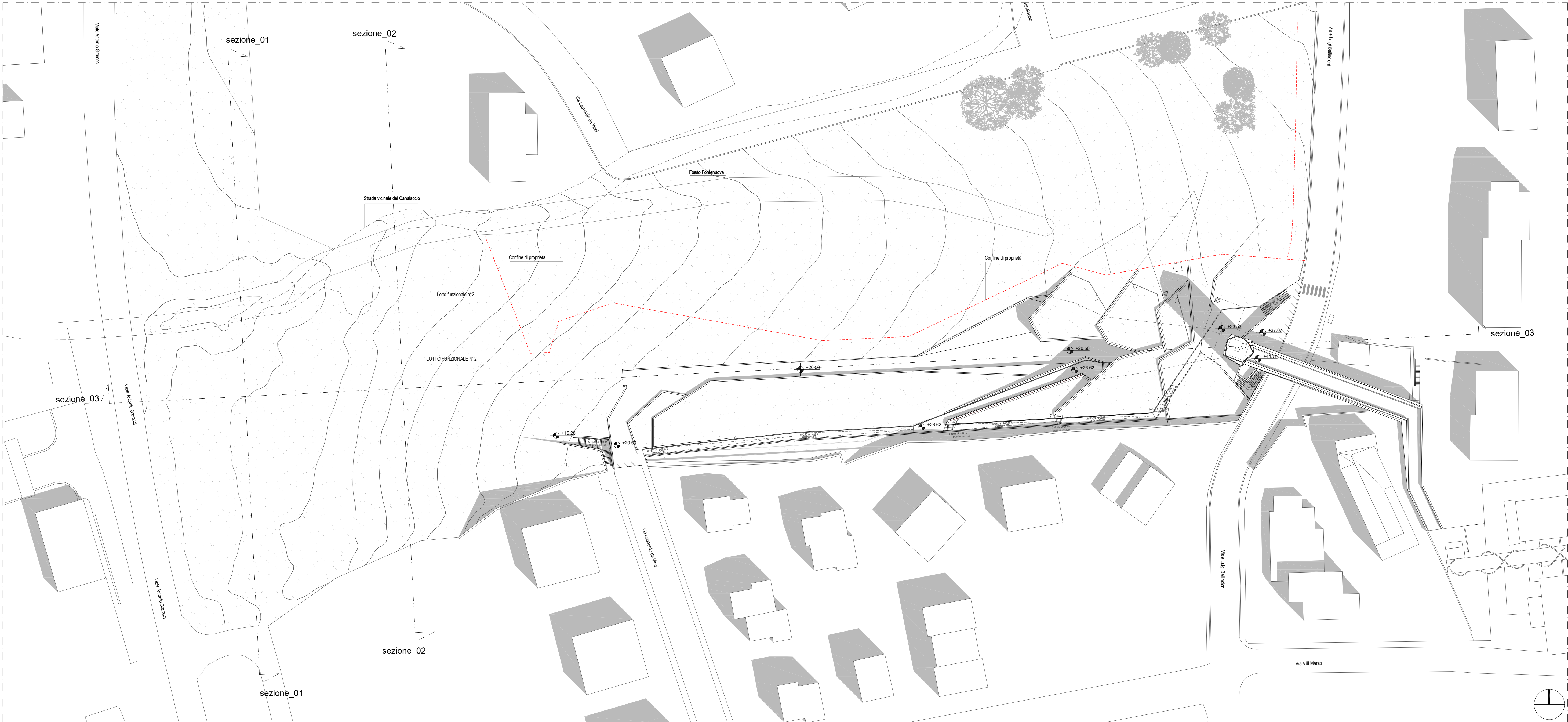
PLANIMETRIA GENERALE Scala 1:500
