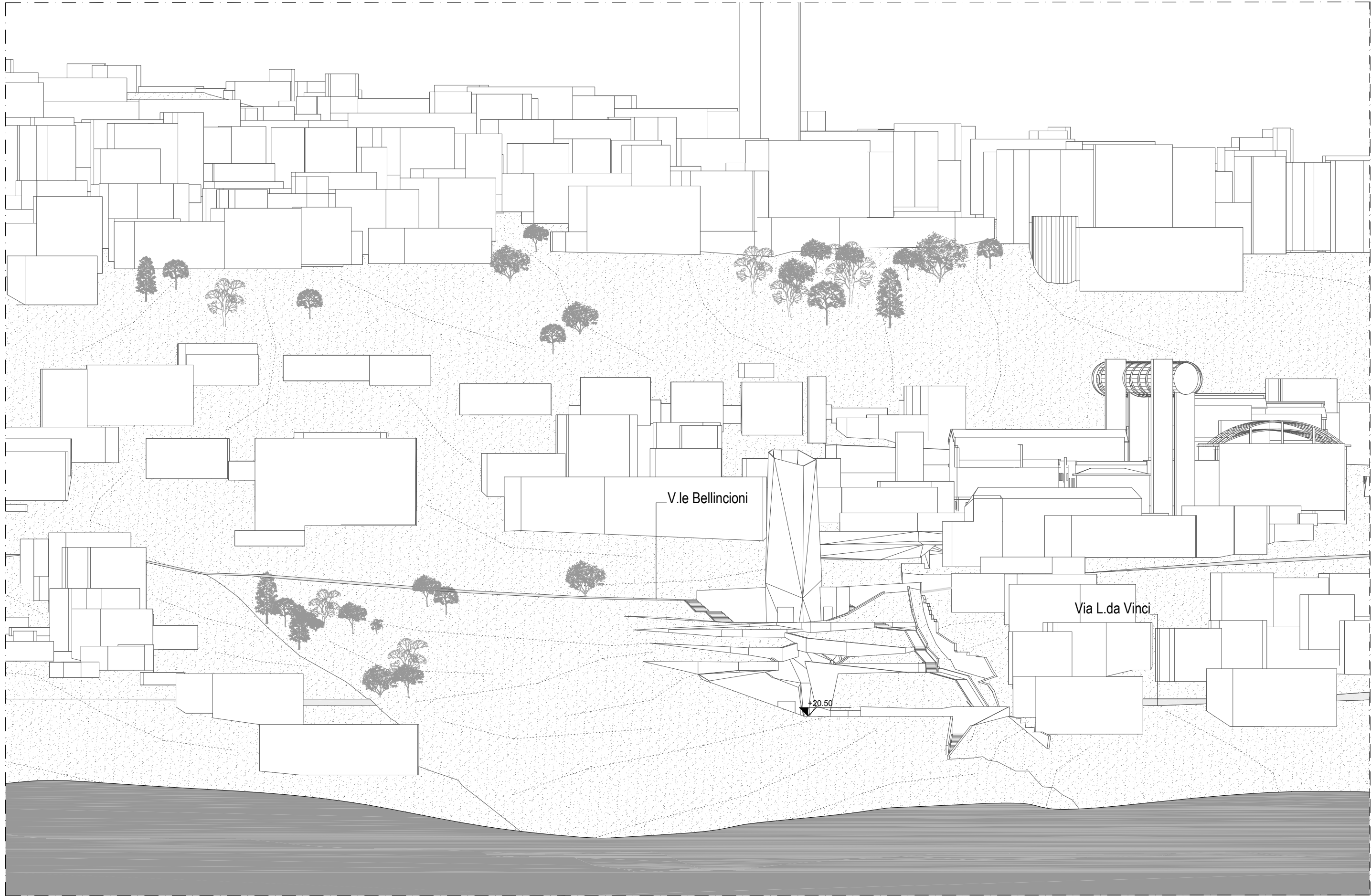
SEZIONE 2-2 Scala 1:500
